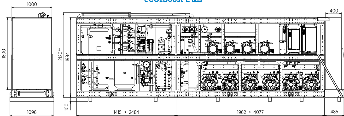
versión para sala de máquinas eCO2Boost L MR
